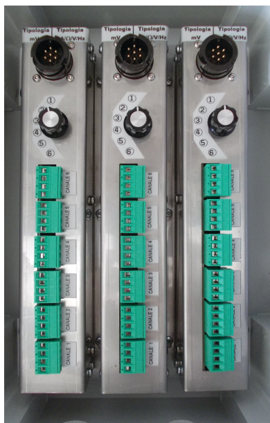
Шкаф с 3 панелями централизации (18 инструментов)
